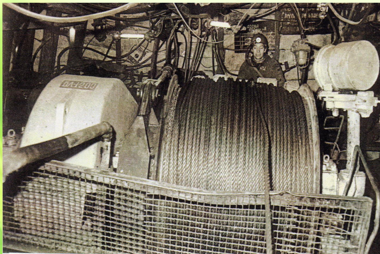
Лебёдка для поднятия и спуска груза.
